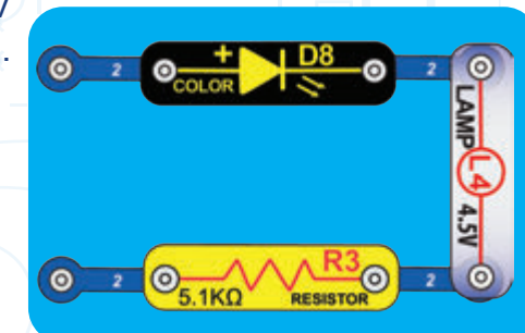
Príklad obvodu zapojeného v sérii
