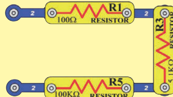
Sériový obvod
