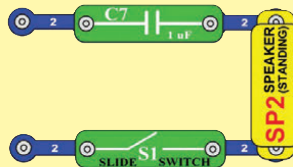
Sériový obvod
