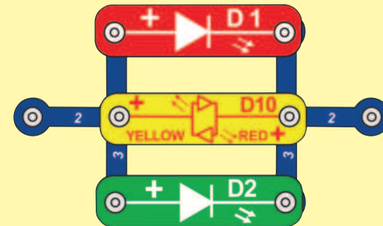
Párhuzamos Áramkör
